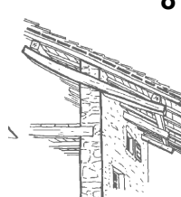
Débord à poutres à bascule
